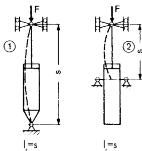
Euler – případ 3
