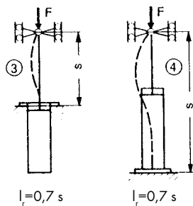
Euler – případ 4
