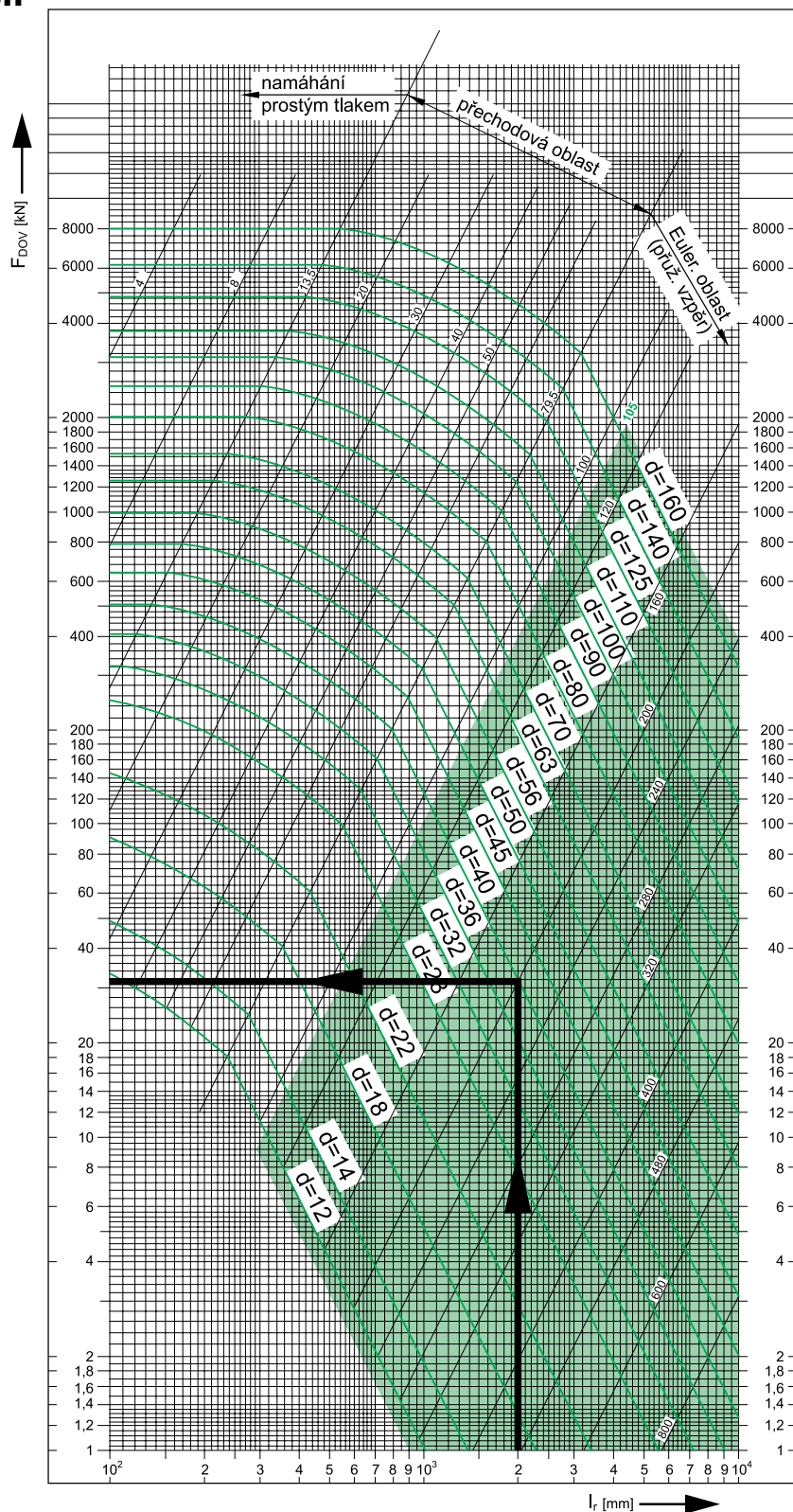
Euler – případ 1
